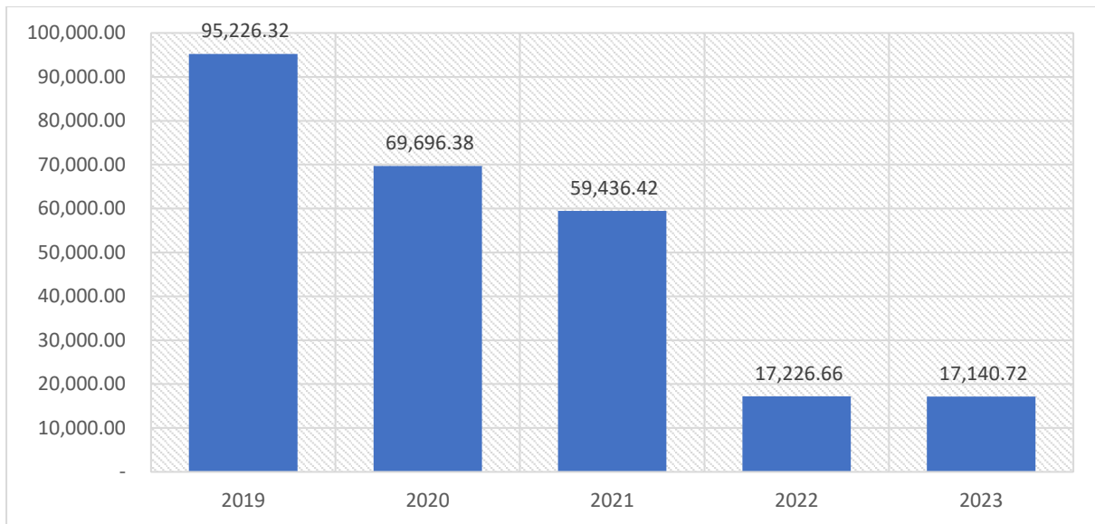
Gambar II.18 Tren Emisi GRK kabupaten Bengkulu Tahun 2019-2023 (Gg CO2 eq)
